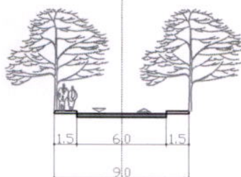
presjek 4-4
