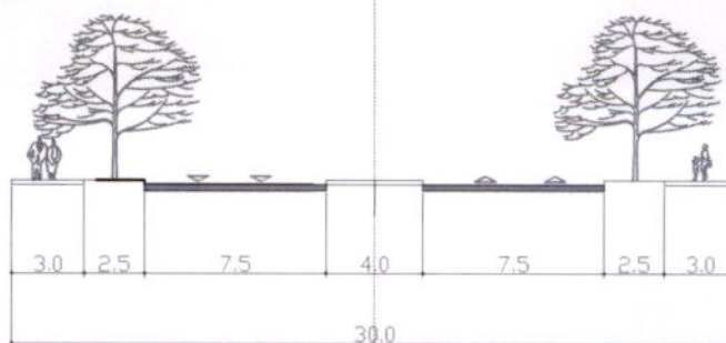
presjek2-2
