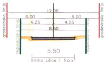
presjek K-K
