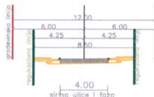
presjek N-N
