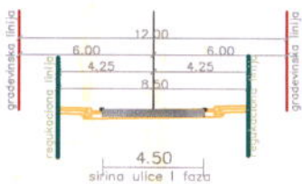
presjek L-L
