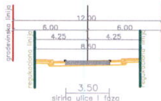
presjek O-O
