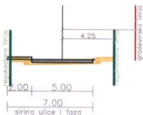
presjek E-E
