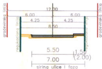
presjek G-G
