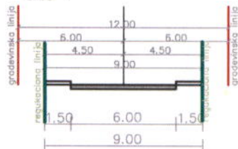
presjek C-C
