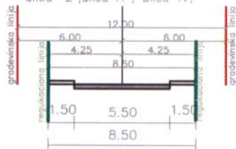
presjek D-D
