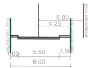
presjek E-E
