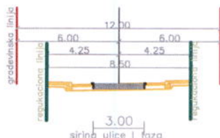
presjek P-P
