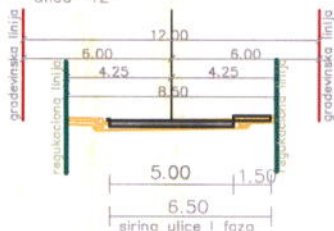
presjek H-H
