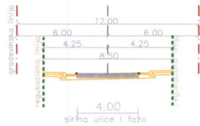
presjek N-N
