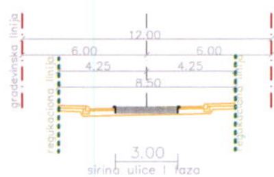
presjek P-P
