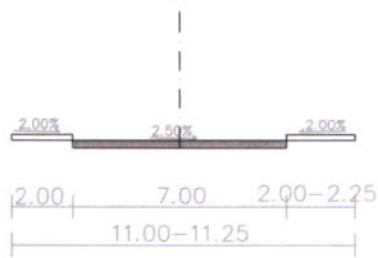
presjek B-B
