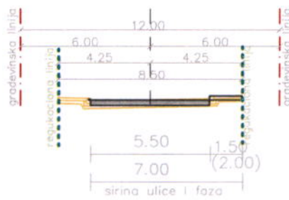
presjek G-G
