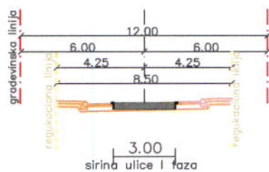
presjek P-P
