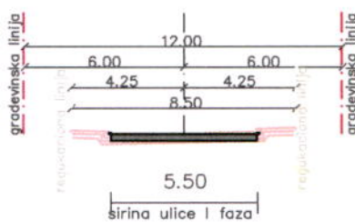
presjek K-K
