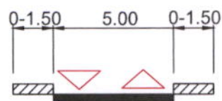
presjek 3 - 3
