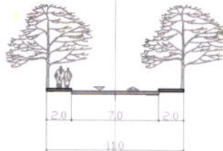
presjek 4-4
