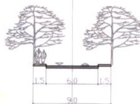
presjek 4-4
