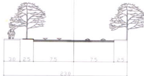
presjek 3-3
