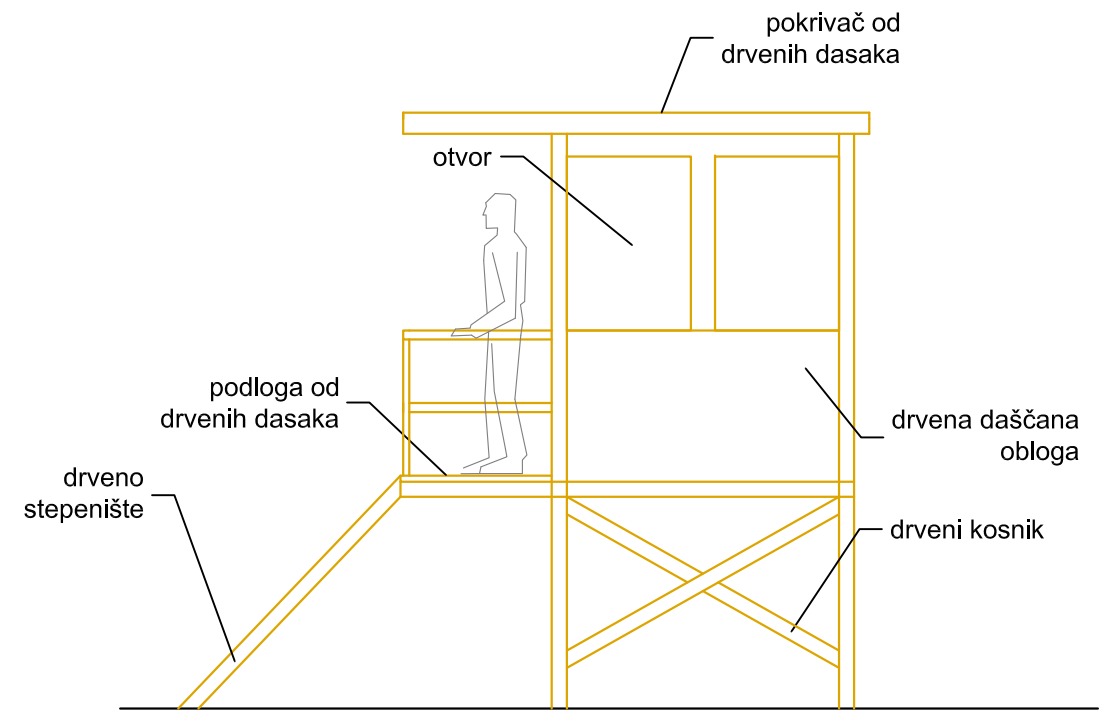
IZGLED A
