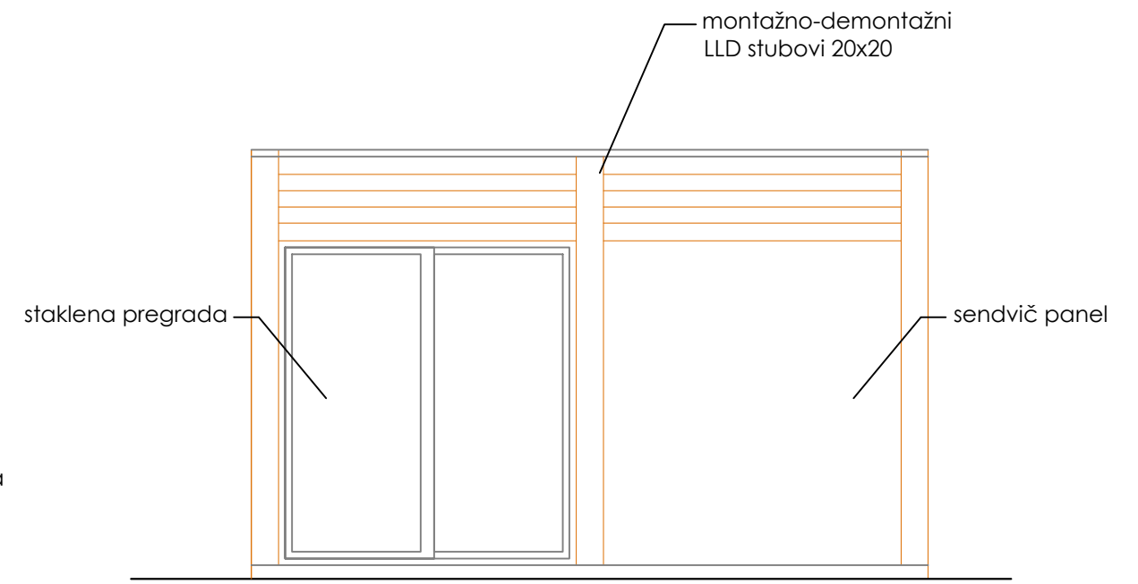
BOČNI IZGLED
