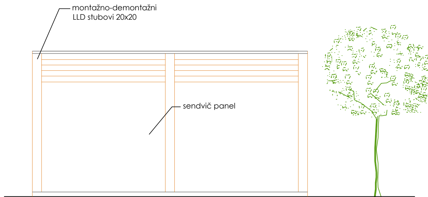
ZADNJI IZGLED
