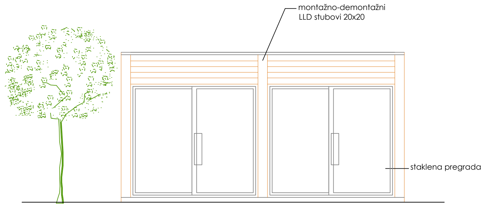
PREDNJI IZGLED
