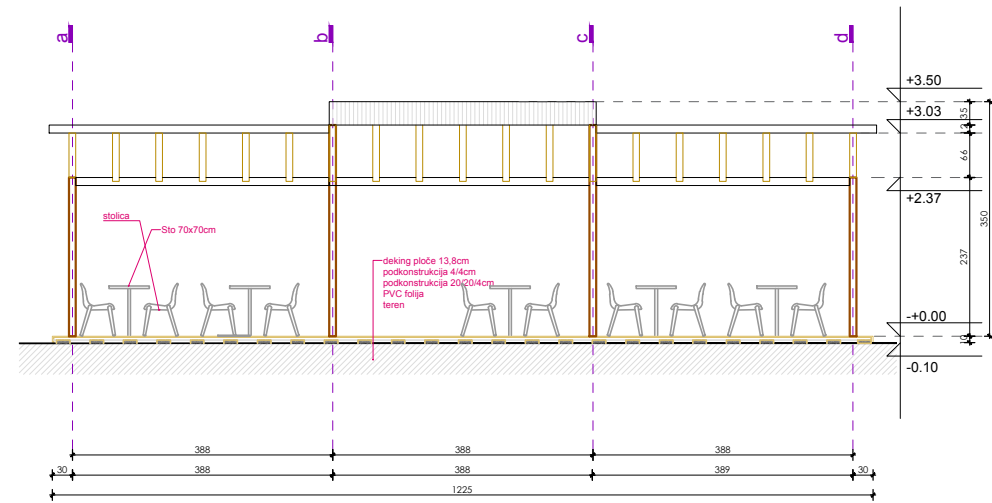
PRESJEK A-A
