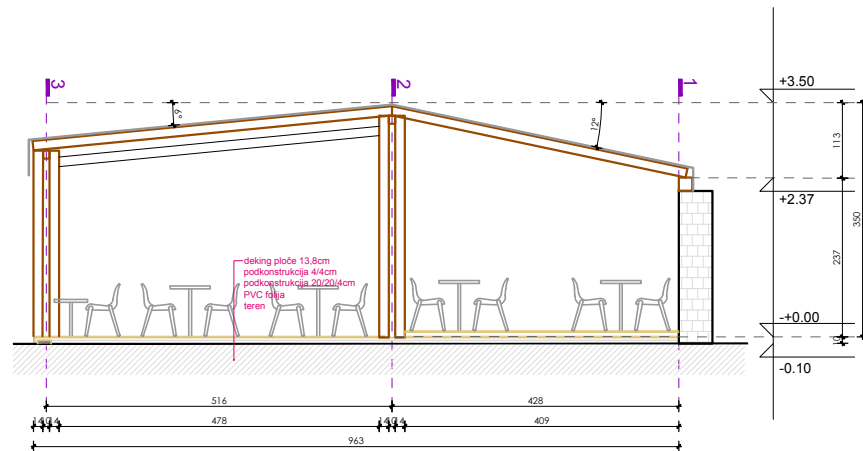
PRESJEK C-C
