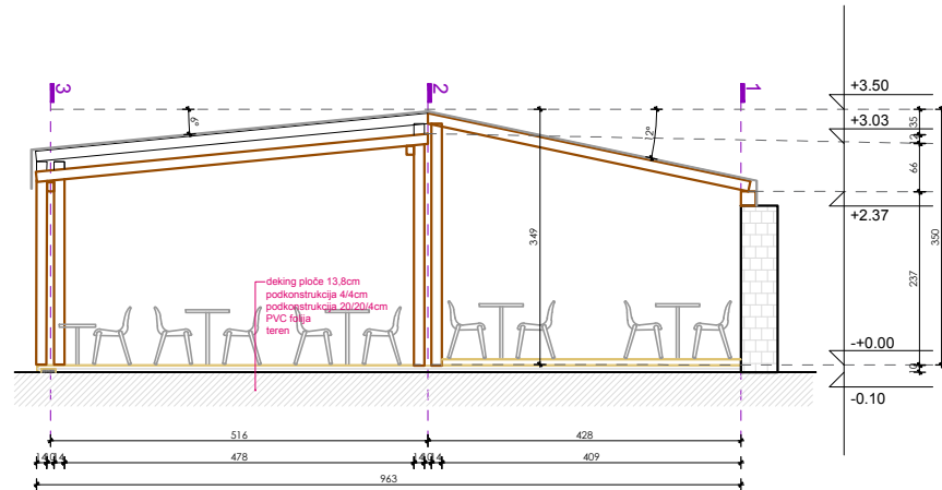
PRESJEK B-B
