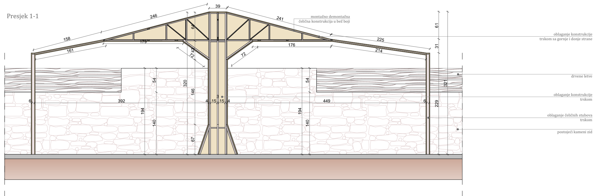
Izgled A-A
