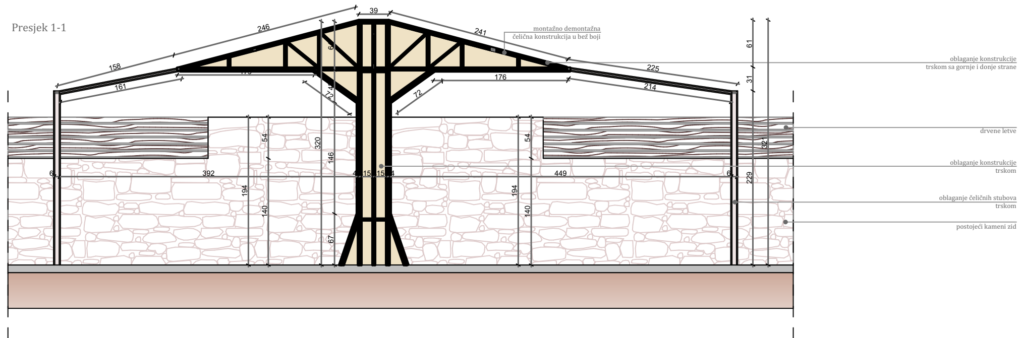
Izgled A-A
