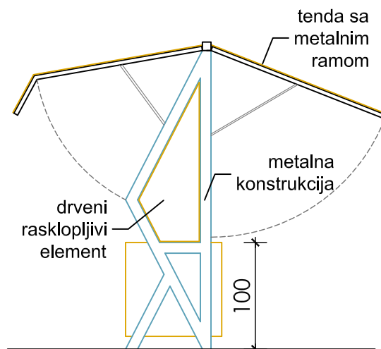
BOČNI IZGLED
