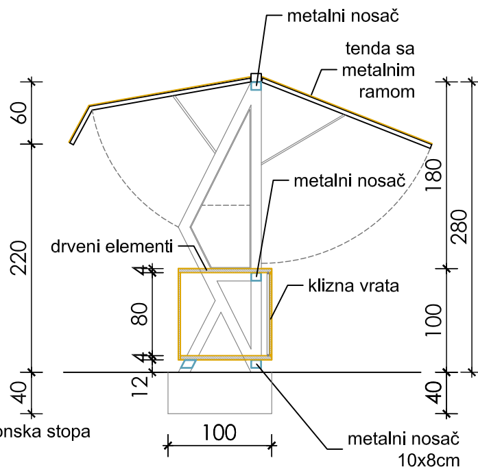
POPREČNI PRESJEK
