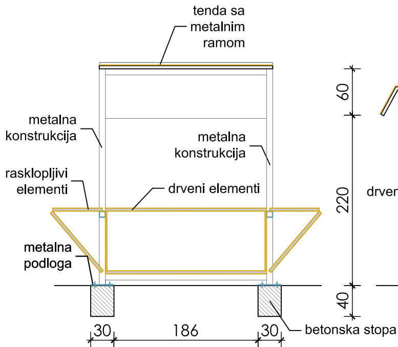
PODUŽNI PRESJEK
