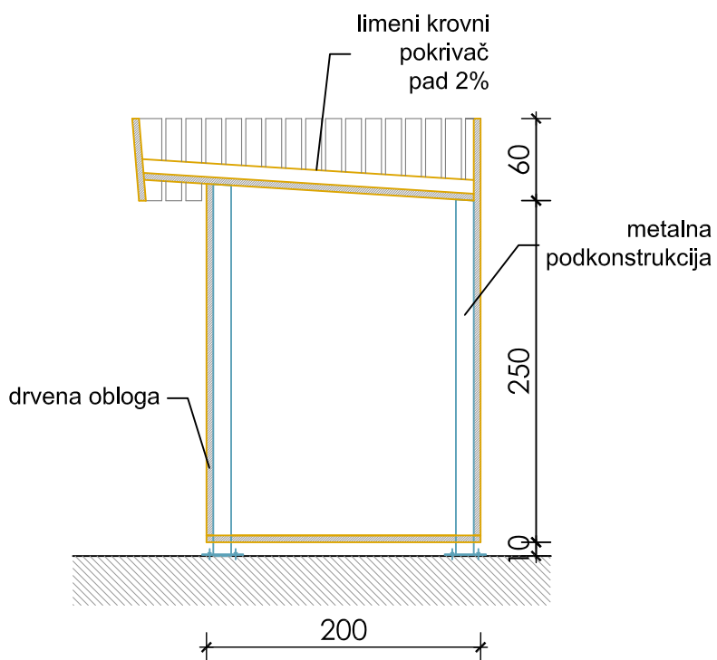
PRESJEK
