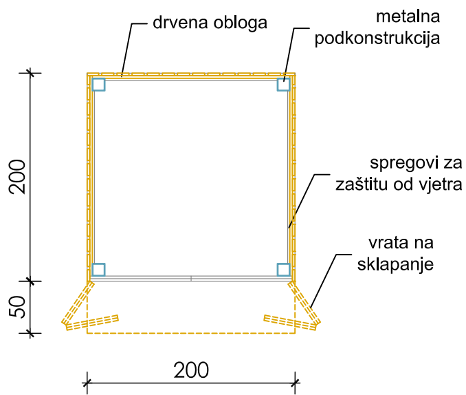
OSNOVA
