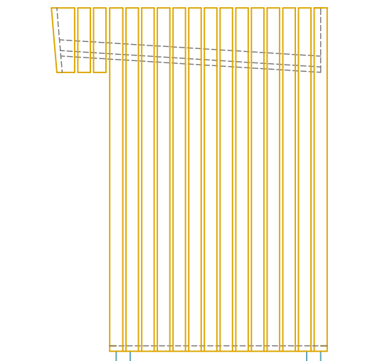
BOČNI IZGLED
